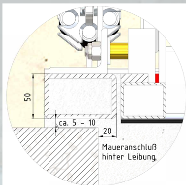
Maueranschluß hinter Leibung
