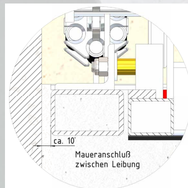
Maueranschluß zwischen Leibung
